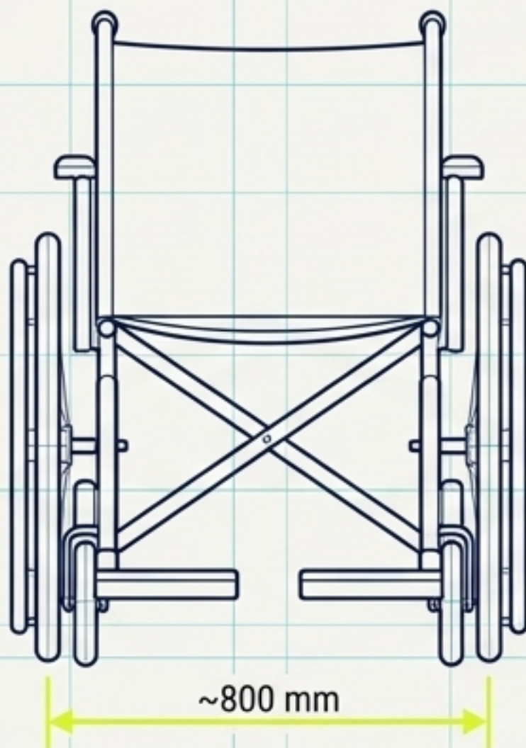
Xe lăn thông thường: Chiều rộng cơ sở ~800 mm. Bánh xe thẳng đứng.
