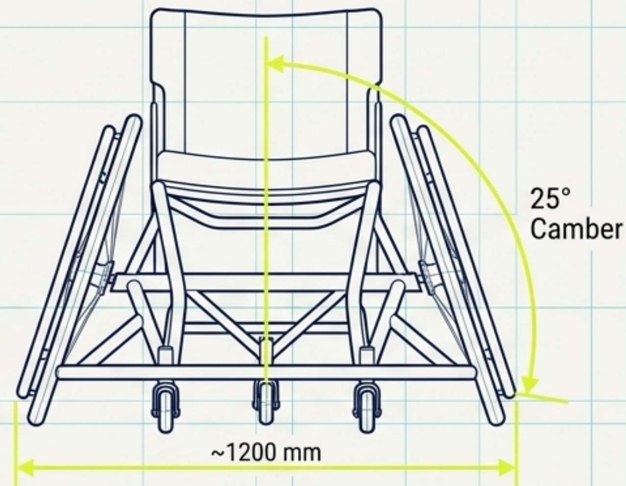
Xe lăn thể thao: Góc nghiêng bánh xe (Camber) lên tới 25°. Tạo ra vùng chuyển động linh hoạt nhưng đòi hỏi bề mặt tựa rộng hơn.
